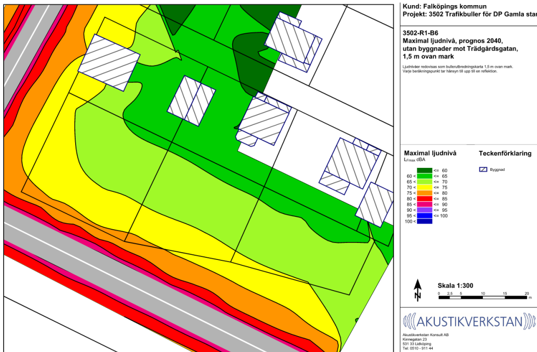
Bild 22 visar maximal ljudnivå vid ny bebyggelse, 1,5 meter ovan mark.
