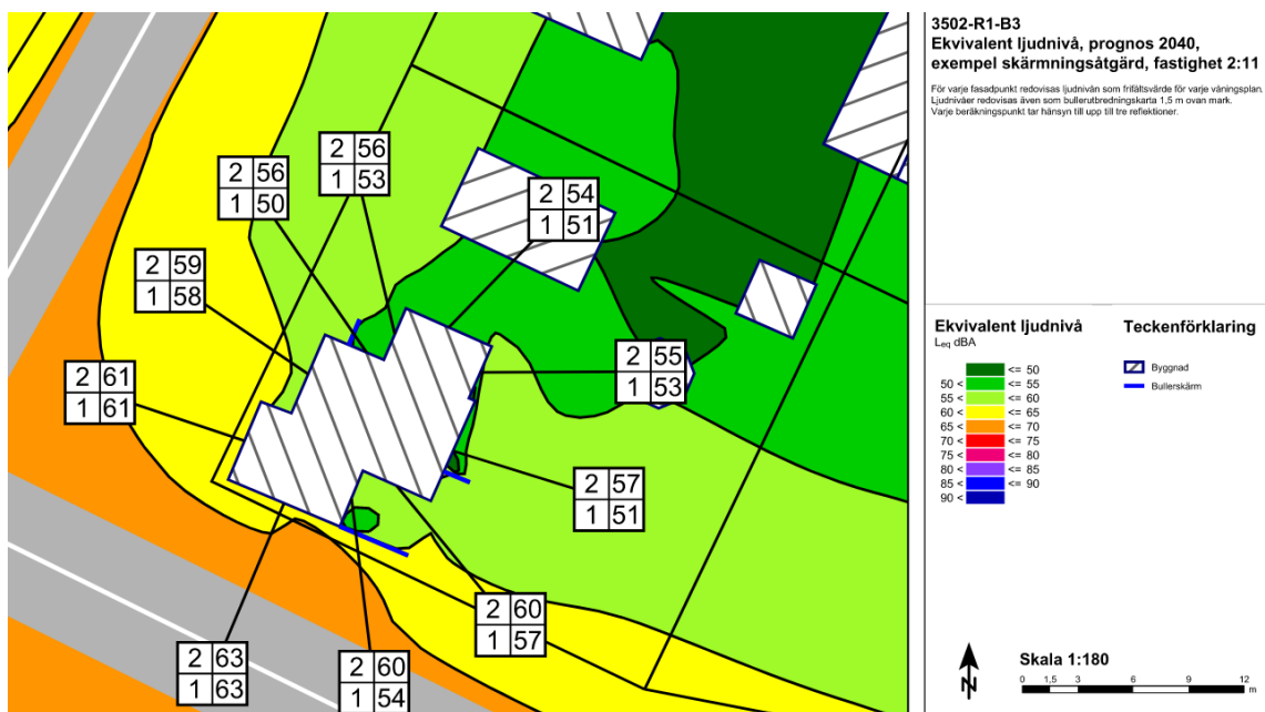
Bild 19 visar ekvivalent ljudnivåer i befintligt läge efter byggnation av bullerskärmar (siffran i nedre rad visar ljudnivån på bottenplan).
